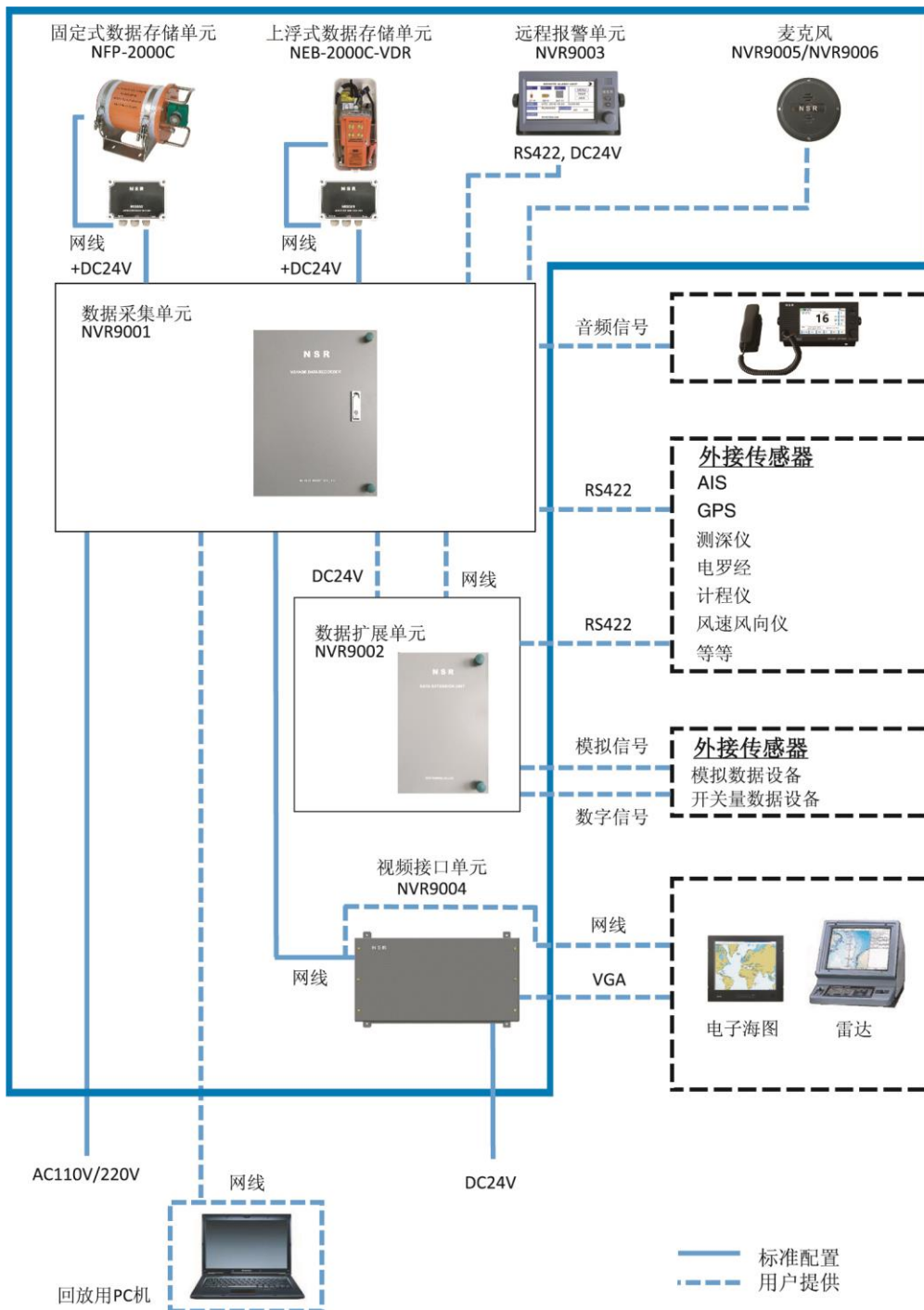
系统框图
