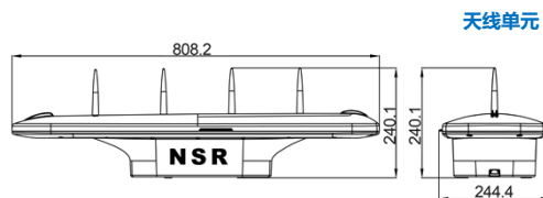
天线单元
