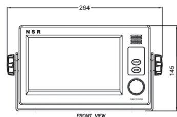
DISPLAY UNIT
